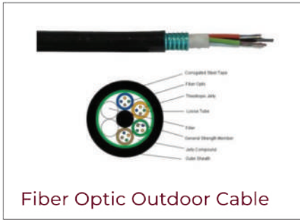
Cable
